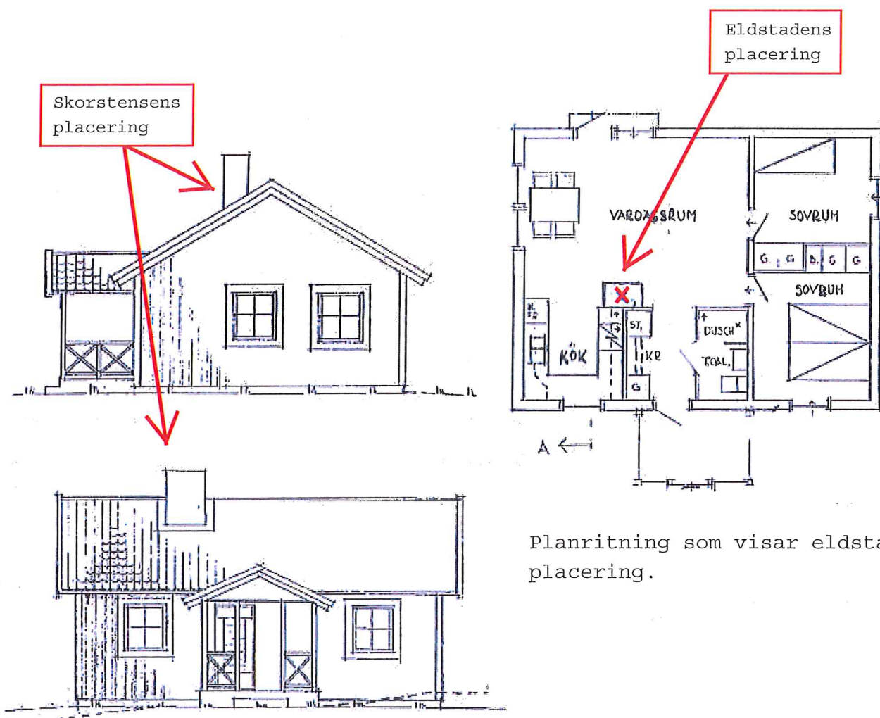
Fasadritningar som visar skorstenens läge.
